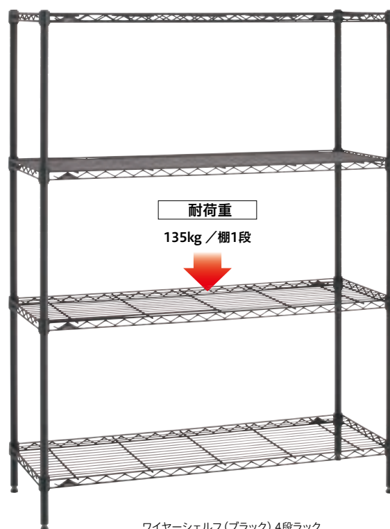
ワイヤーシェルフ (ブラック) 4段ラック 外寸 : W1200×D450×H1600mm
